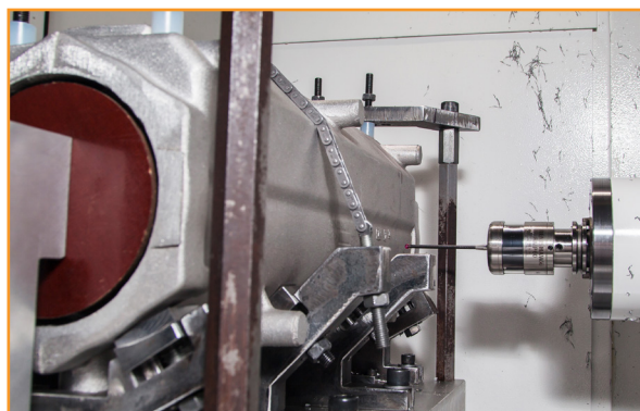
Samodejno nastavljanje obdelovancev s sistemom RMP60
