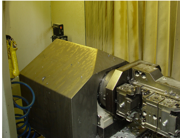
Bezdotykowy laserowy system Renishaw zainstalowany poza przestrzenią roboczą obrabiarki
