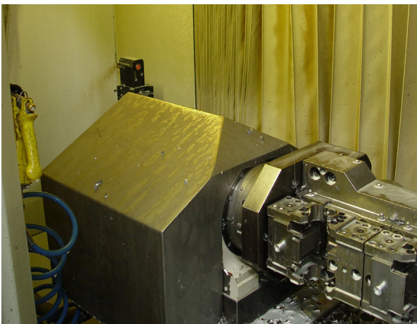
機械の加工範囲の外側に取り付けられたレニショーの非接触式レーザーシステム
