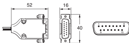
Connettore di tipo D a 15 pin (codice di terminazione D, L)
