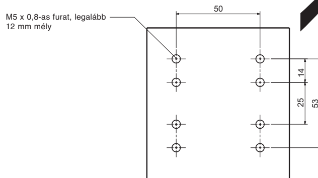
A TÍPIKUS FELERŐSÍTÉSI FELÜLET MEGMUNKÁLÁSI RAJZA
