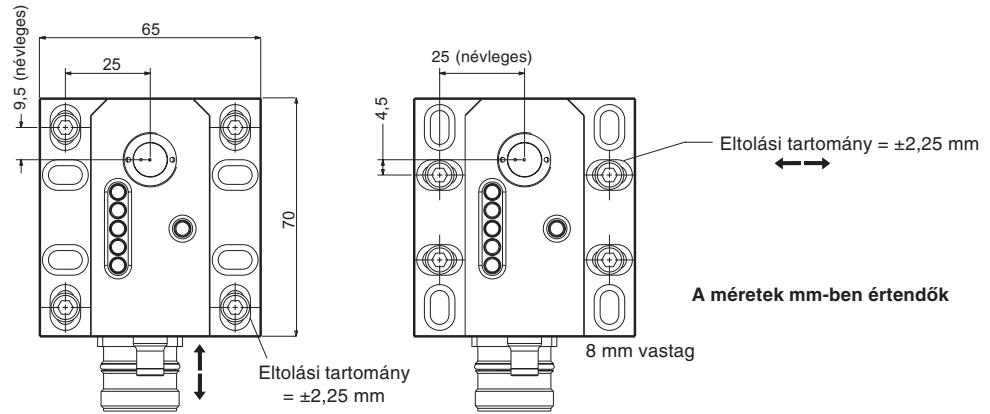
A FELERŐSÍTŐ LEMEZ RÉSZLETRAJZA
