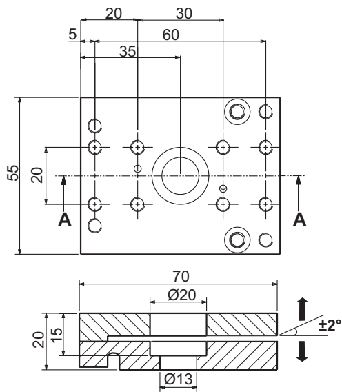
A-A METSZET
