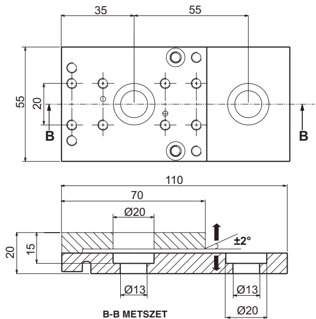
B-B METSZET
