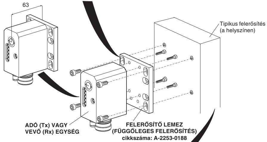
A FELERŐSÍTŐ LEMEZ RÉSZLETRAJZA
