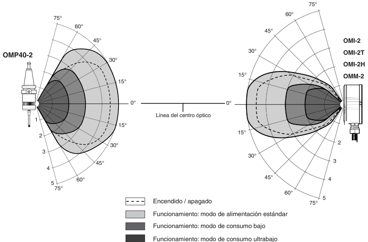
Gráfico típico a +20 °C. Alcance de transmisión en m
