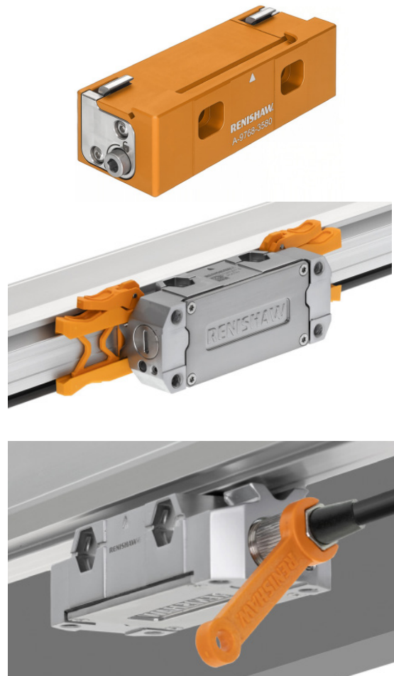
Figure 5. Exemples d'accessoires d'installation (FORTiS-S illustré)
