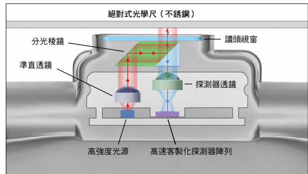
圖 1. FORTiS 光學尺讀頭的光學鏡組示意圖
