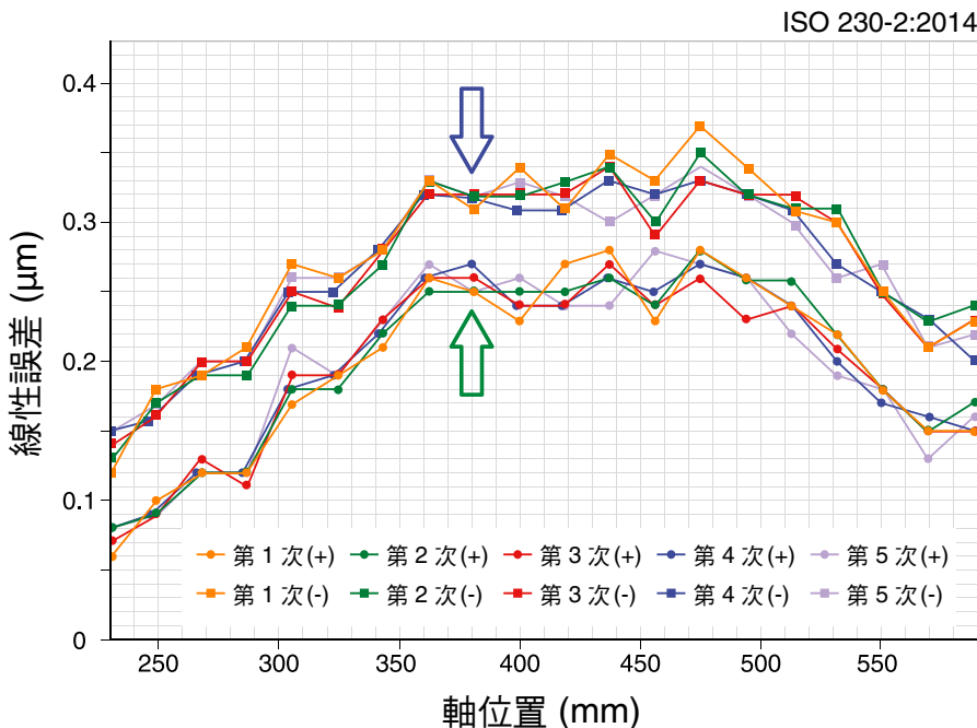
圖 2. 在五次試驗的執行中，FORTiS 光學尺的正向（前進）和負向（後退）滯滯誤差
